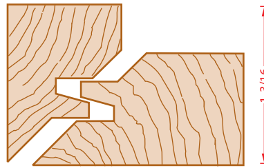
55390 45°
