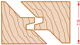
55389 45°
