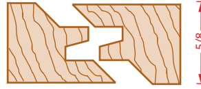
55391 45°
